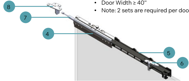
CLAMP OPTION A: SOFT-CLOSE
